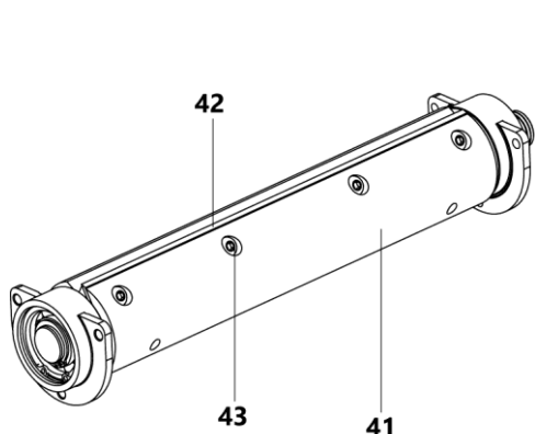
Рисунок 6. Общий вид ножевого вала 41 – вал ножевой; 42 – нож; 43 – винт зажимной
